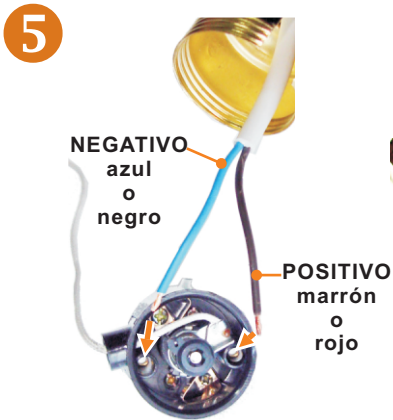
Pasar los cables a través de los taladros, respetando la polaridad indicada. Manipular con cuidado para que no salte el muelle del interruptor.
