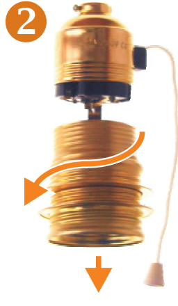
Desmontar el portalámparas, según indican las figuras
